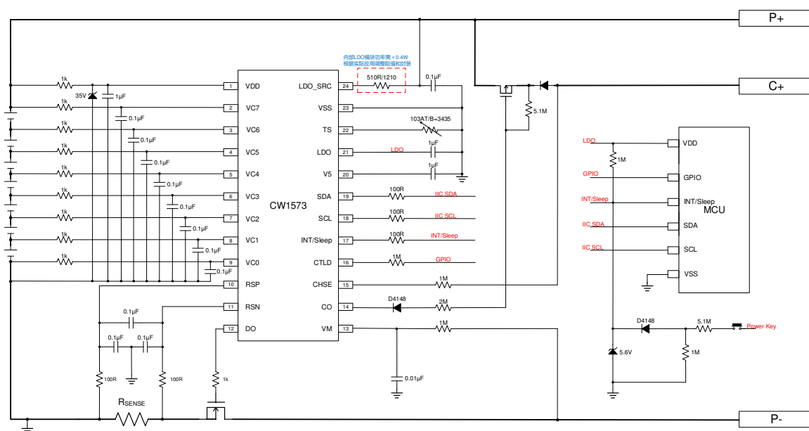
7 串应用电路 (CH+)
