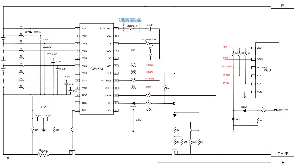
7 串应用电路（同口/CH-）
