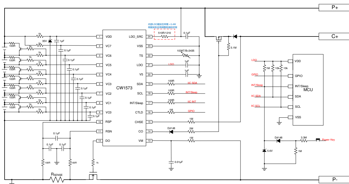
7 串带均衡应用电路 (CH+)
